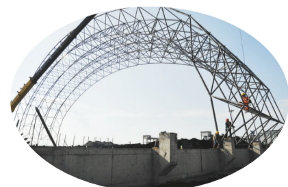
广纳煤焦化物料堆场覆盖工程建设中
