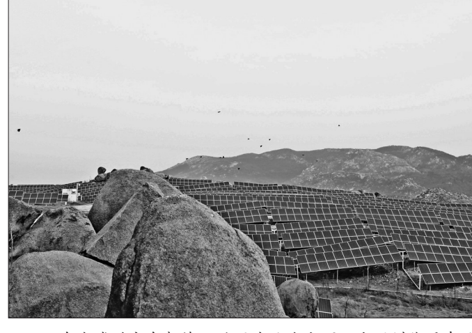
山东省滕州市东郭镇20兆瓦光伏发电项目由深圳能源有限公司投资建设,占地1000亩,是利用荒山建设的节能环保项目。从2015年底投产以来,已累计发电2400万度,大约相当于节约标准煤0.77万吨,减排SO 2 600吨、CO 2 1.994万吨、粉尘0.544万吨、氮氧化物300吨。
