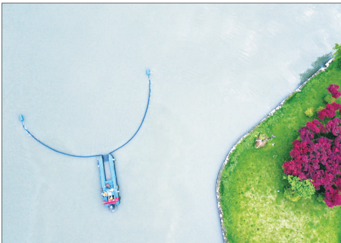
近日，浙江省温州乐清市城南街道针对辖区河道实际情况，投入使用新能源漂浮物智能清理船清理水面垃圾。该船围栏可自动化遥控作业，能聚拢水面3米—30米范围内的各种漂浮物，每小时可清理10万平方米水面，靠岸后可“一键”完成垃圾沥干出卸，大大提高水面保洁效率。
